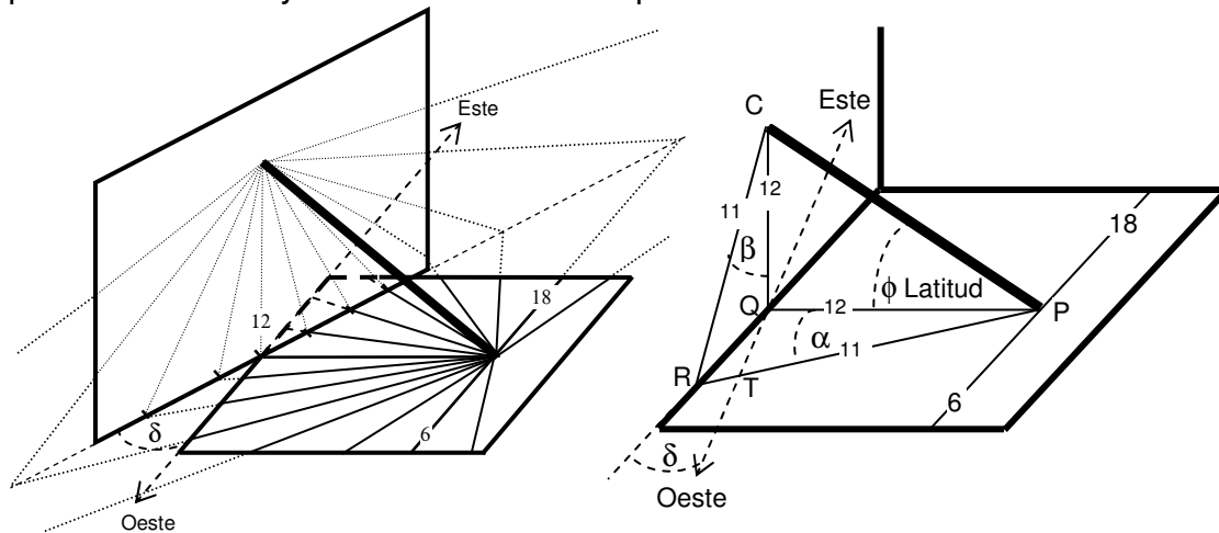
Figura 5: Trazado de un reloj vertical declinante por el método gráfico y el planteamiento trigonométrico
