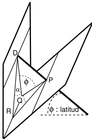
Figura 3: Relaciones trigonométricas
